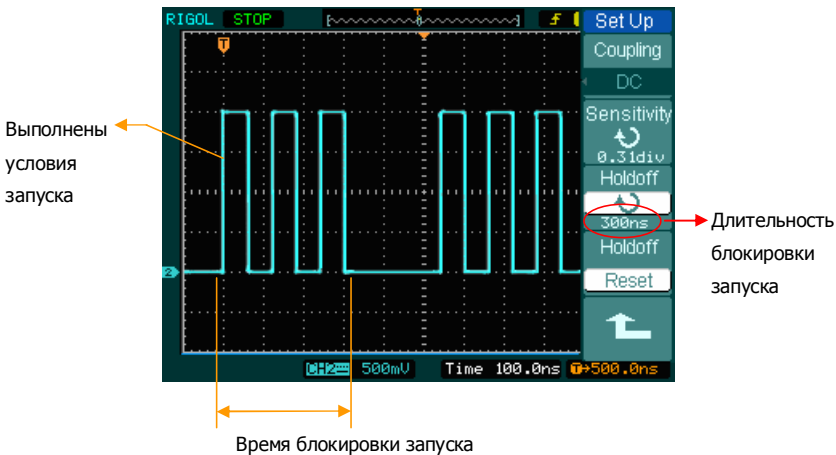
Рисунок 2-65. Блокировка запуска
