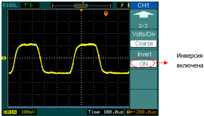
Форма сигнала после инверсии
