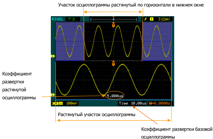
Рисунок 2-39. Окно увеличения фрагмента
