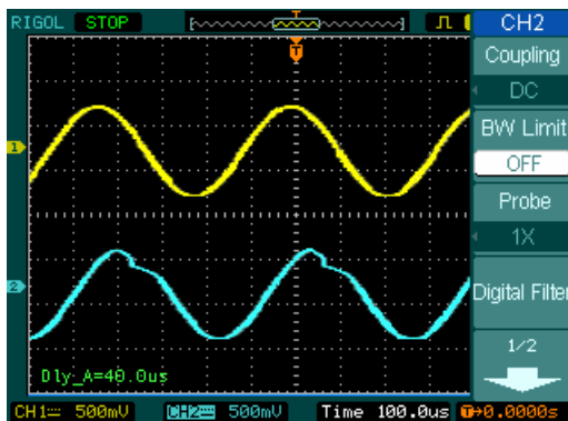
Рисунок 3-1. Измерение задержки между сигналами
