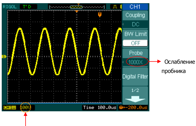
Вертикальный масштаб Вольт/дел.
