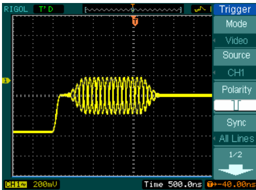
Рисунок 2-48. Запуск по видеосигналу: синхронизация по строке
