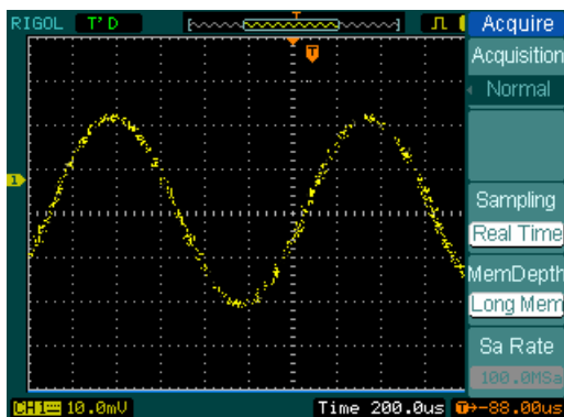
Рисунок 2-68. Сигнал, содержащий шумы, обычный режим регистрации.
