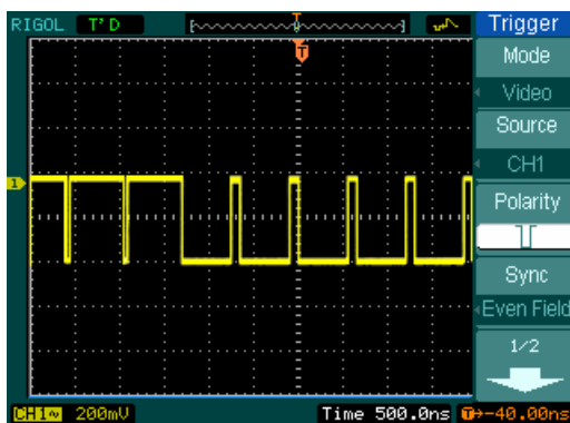
Рисунок 2-49. Запуск по видеосигналу: синхронизация по полю
