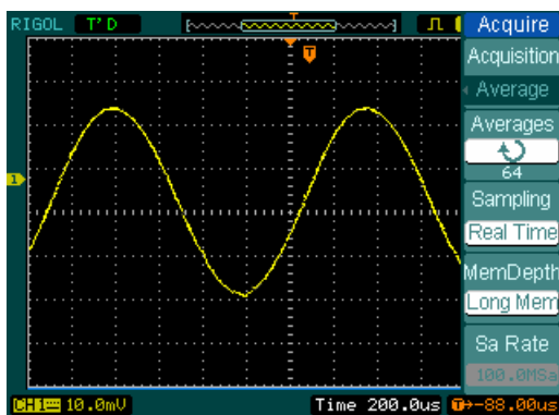
Рисунок 2-69. Сигнал, содержащий шумы, режим усреднения
