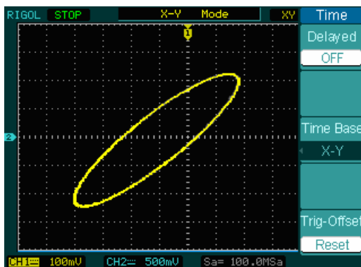
Рисунок 2-40. Вид экрана для режима X-Y
