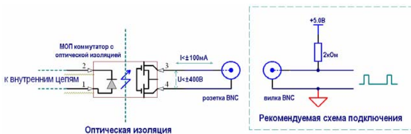
Рисунок 2-99. Схема выхода Pass/Fail и подключение к нему.
